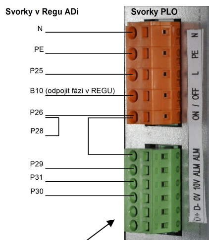
Elektrické zapojení s REGU ADi
