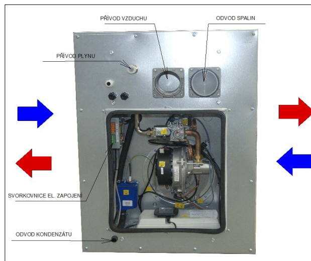
Čelní strana plynového ohřívacího modulu PLO
